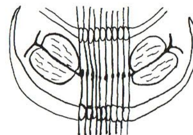
Tek 2: Sporenkegels bij Calamites De stam was evenals de huidige paarden-
