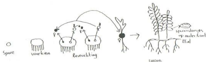
Tekening 1: de voortplanting van sporenplanten.
