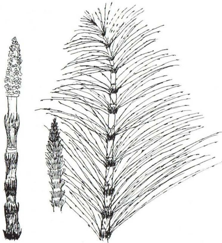
Tekening 3: Van sporenaar tot groene stengel
